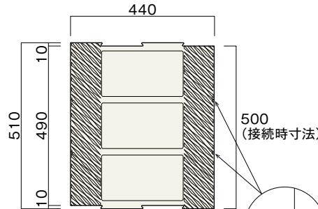
510×440×1~7(スローブ形状)
